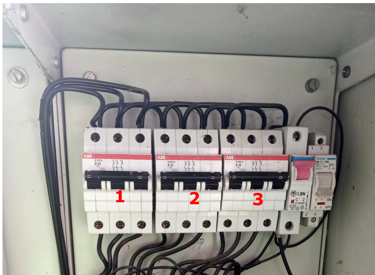
Obr. 3 Detail RVO-1 s vyznačenými větvemi
